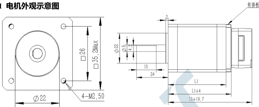
图 6.1 ISS35 系列一体机外观示意图
