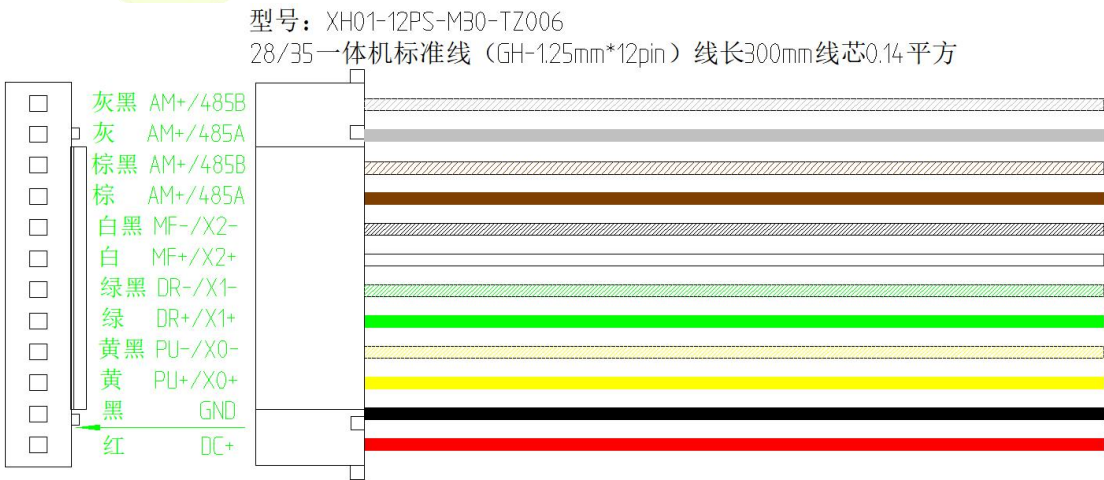
图 6.2 ISS35 系列配线示意图
